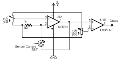
Gambar 2. Rangkaian Kondisi Sinyal Sensor Cahaya
